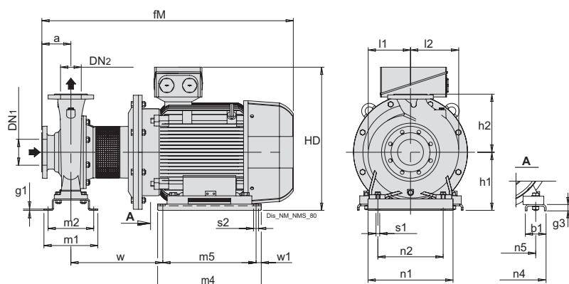
Brides EN 1092-2
