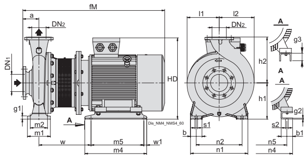
Brides EN 1092-2
